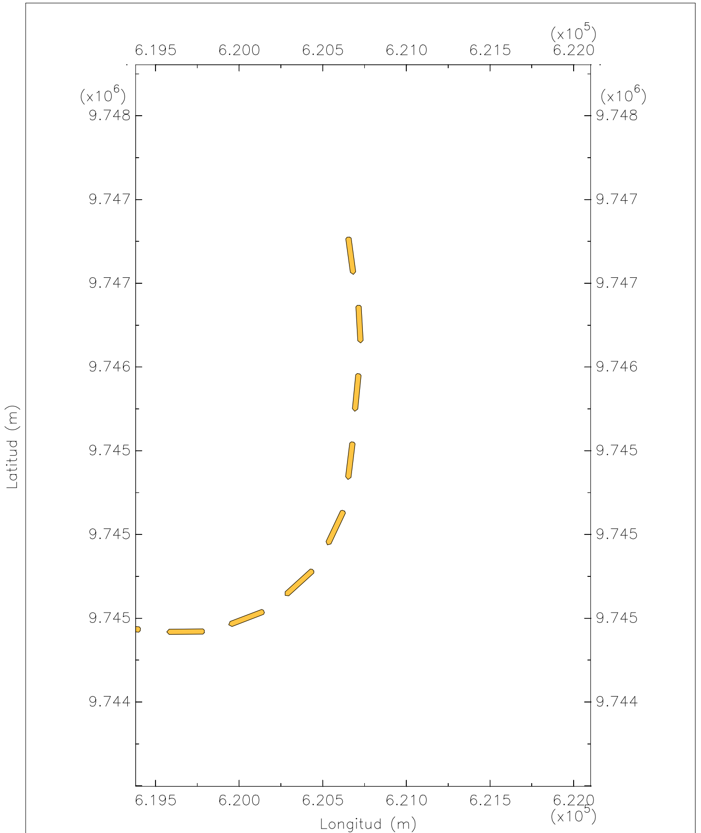
Z3T1 Trayectoria del barco granelero
