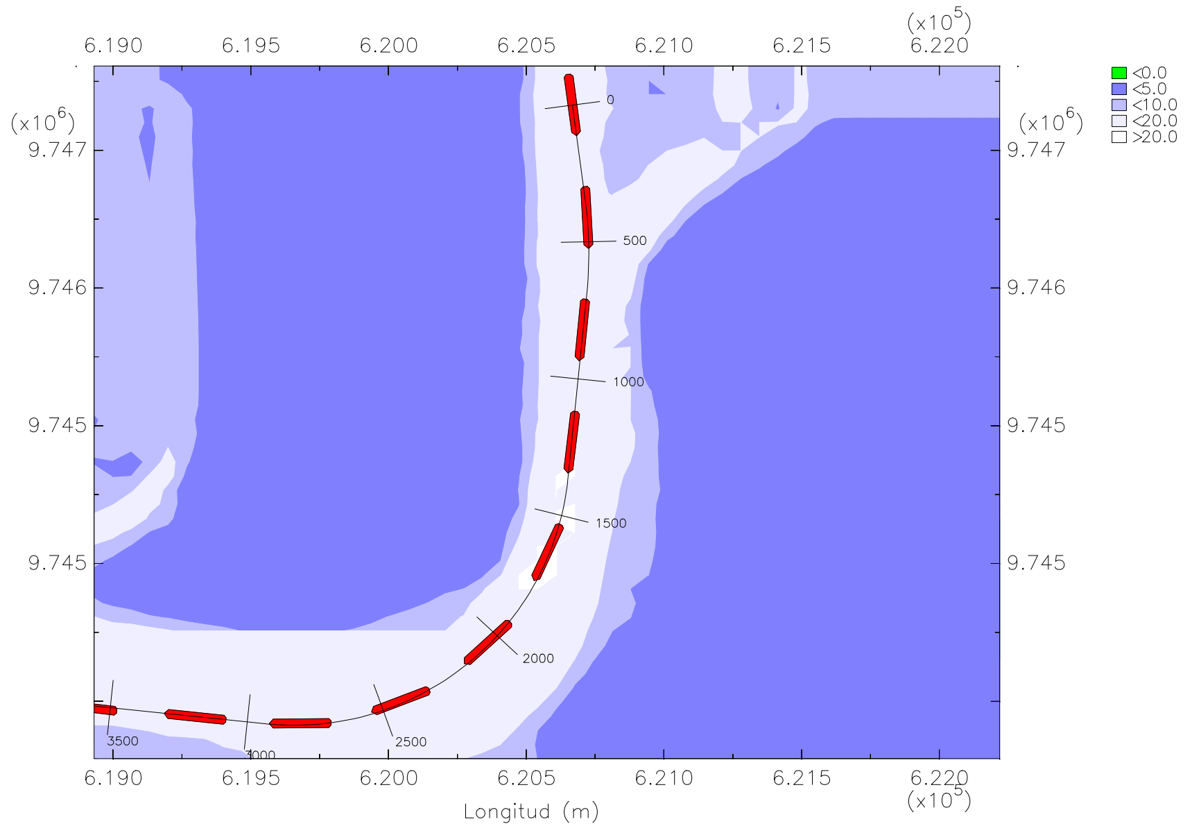
Z3T1 Trayectoria del barco granelero en reflujos
